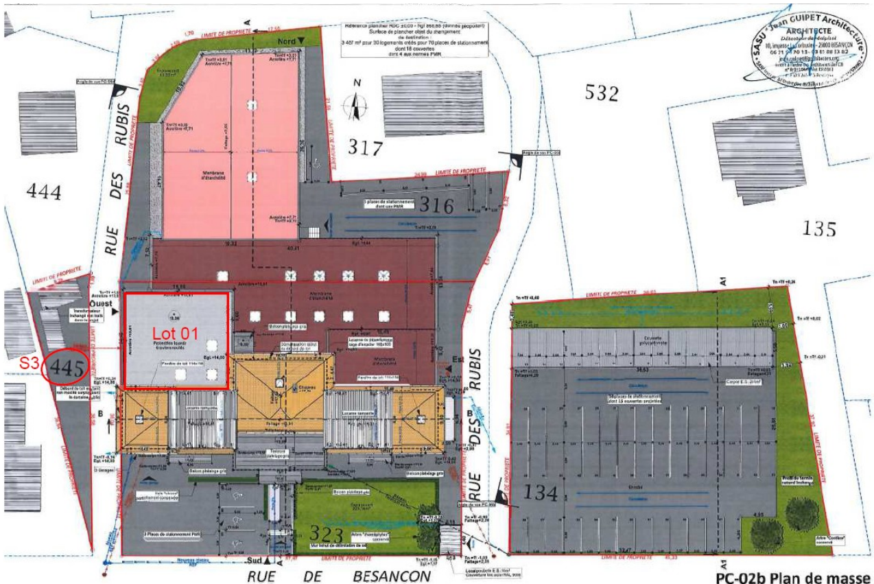
PC-02b Plan de masse 1:300
